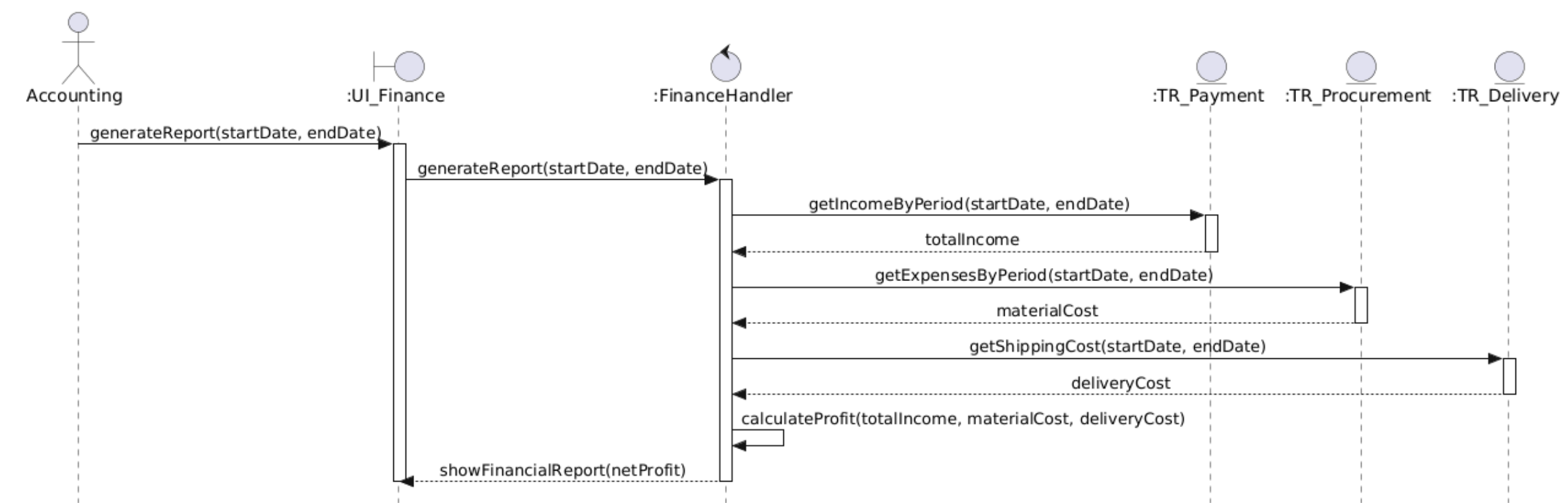
Sequence Diagram: Mengelola Laporan Keuangan
