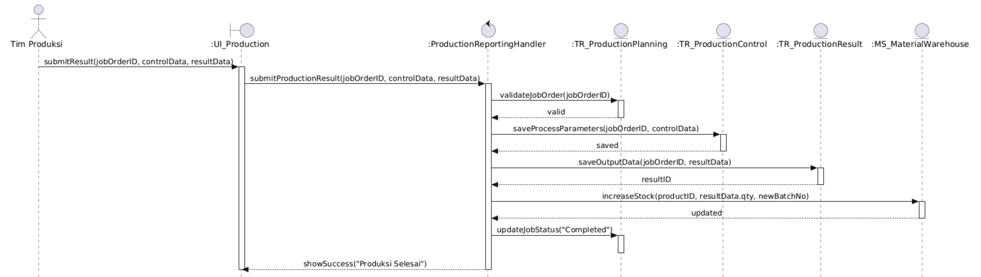
First Cut Sequence Diagram : Membuat Laporan Produksi
